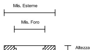
PROSPETTO/SEZIONE CHIUSINO
