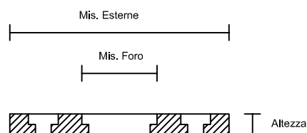
PROSPETTO/SEZIONE COPERCHIO
