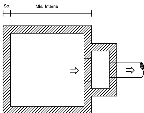
PIANTA POZZETTO
